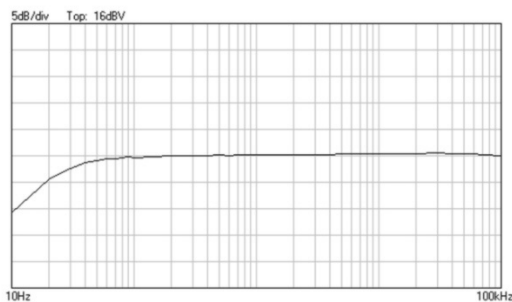
Respuesta en frecuencia @ 8 ohm
